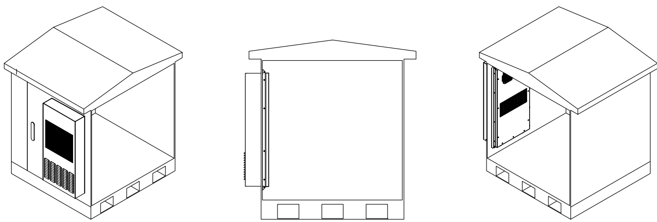
安装图示/Installation Diagram
